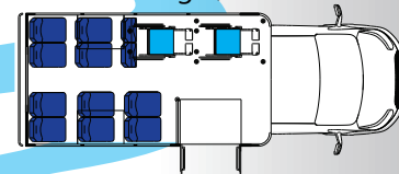
10+2 Passenger, 2 w/c
