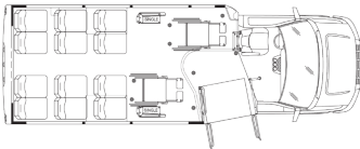
24', 12+2 Passenger, 2 w/c
